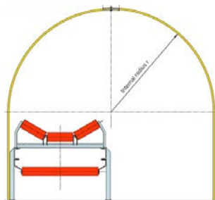
kryty kryjící celý dopravník a lávky
