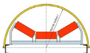
půlkruhové kryty bez rovných bočnic
