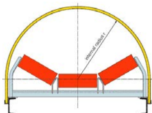
půlkruhové kryty s rovnými bočnicemi
