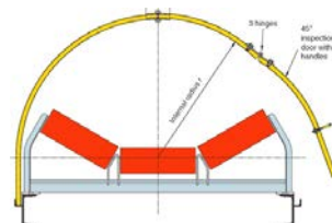
inspekční dveře pro kryty
