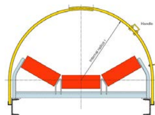
odnímatelné kryty
